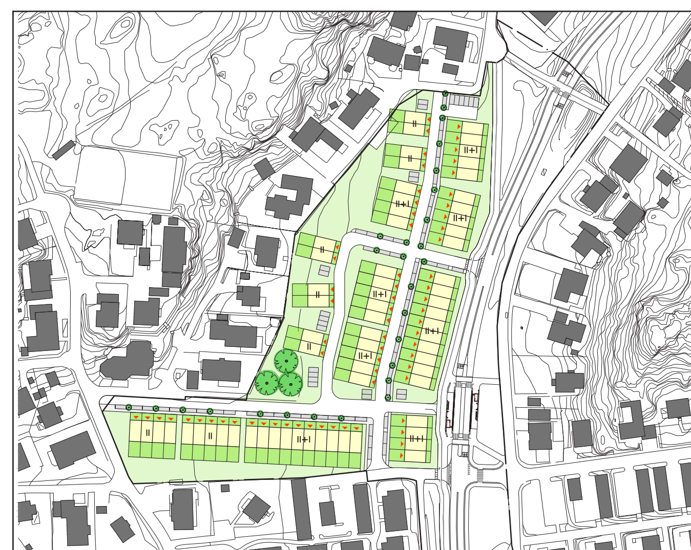
Illustrationsritning för den norra delen av planområdet
