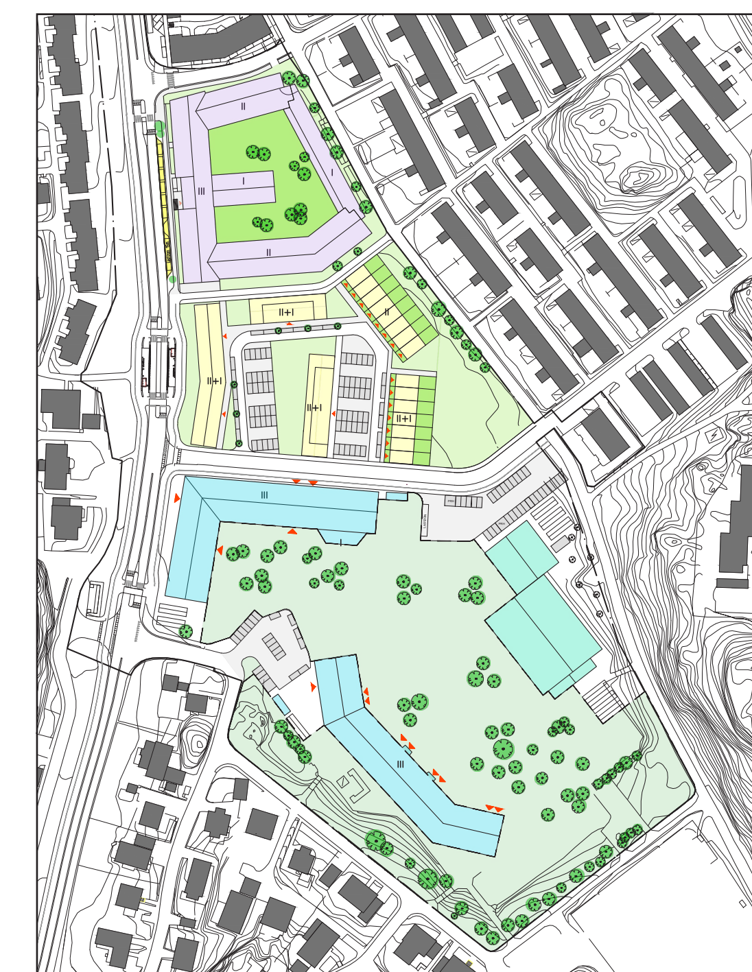
Illustrationsritning för den södra delen av planområdet
